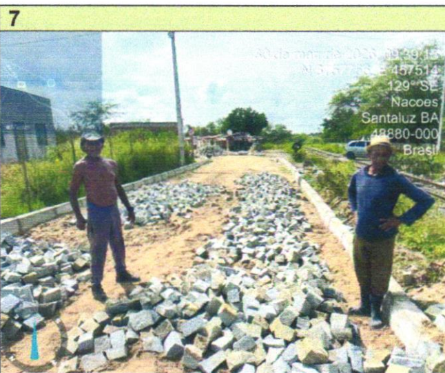
7 DESCRIÇÃO EXECUÇÃO DE PAVIMENTO EM PARALELEPÍPEDOS, REJUNTAMENTO COM ARGAMASSA TRAÇO 1:3 (CIMENTO E AREIA). AF_05/2020
