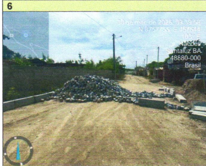
6 DESCRIÇÃO EXECUÇÃO DE PAVIMENTO EM PARALELEPÍPEDOS, REJUNTAMENTO COM ARGAMASSA TRAÇO 1:3 (CIMENTO E AREIA). AF_05/2020
