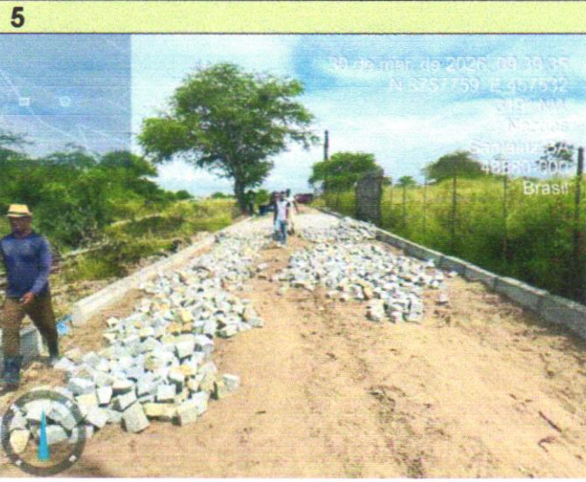
5 DESCRIÇÃO EXECUÇÃO DE PAVIMENTO EM PARALELEPÍPEDOS, REJUNTAMENTO COM ARGAMASSA TRAÇO 1:3 (CIMENTO E AREIA). AF_05/2020
