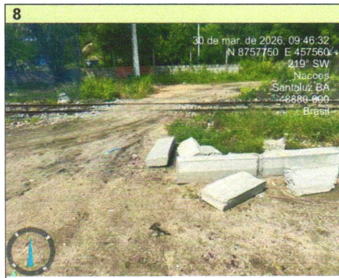
8 DESCRIÇÃO EXECUÇÃO DE PAVIMENTO EM PARALELEPÍPEDOS, REJUNTAMENTO COM ARGAMASSA TRAÇO 1:3 (CIMENTO E AREIA). AF_05/2020
